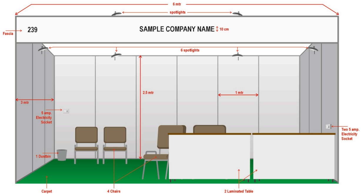
Front Side Open - 18 sq. m. - Depth 3 m. x Front 6 m.
